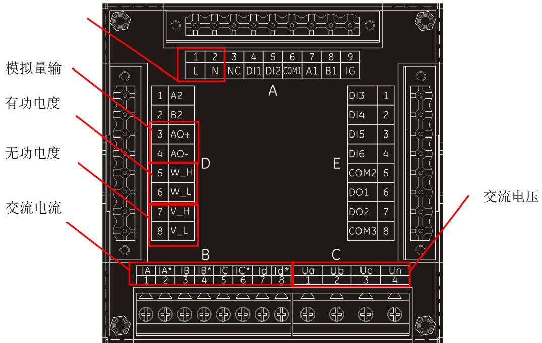
图 3.3 T5 背部端子图
