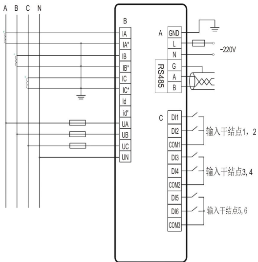
三相四线 CT 输入，电压直接接入
