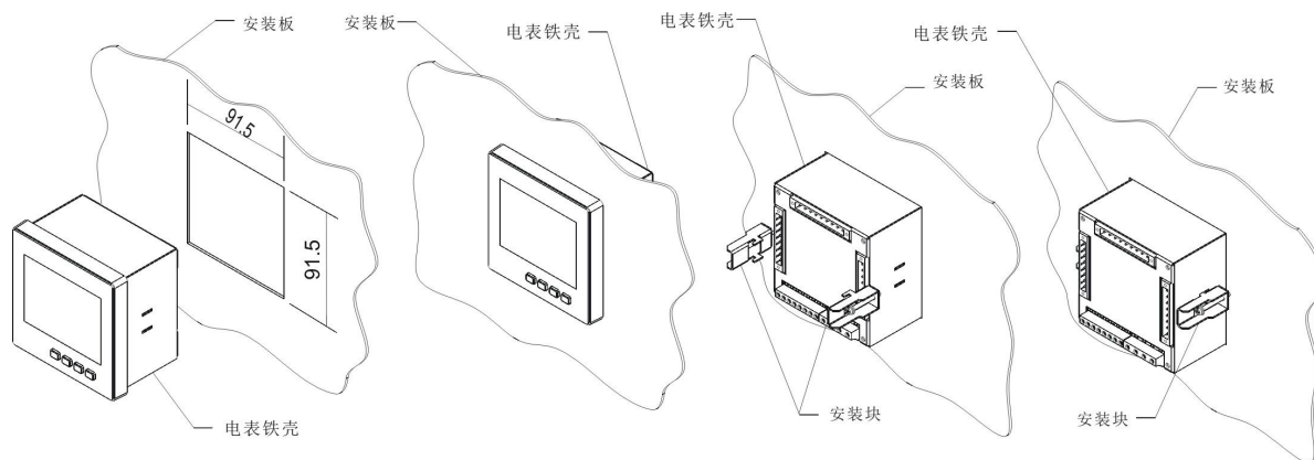
图 3.1 智能多功能仪表安装图
