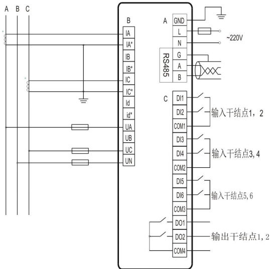
三相三线 CT 输入，电压直接接入
