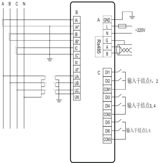
三相四线 3PT、3CT 接线图
