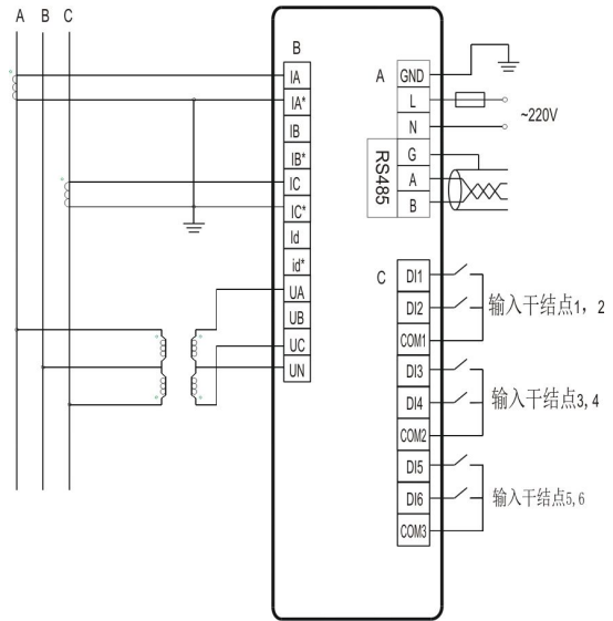
三相三线 3PT、3CT 接线图
