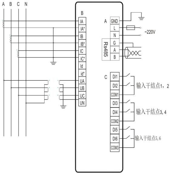
三相四线 3PT、3CT 接线图
